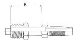
Short pilot "O" ring wartel buitendraad "O" ring male swivel "O" ring écrou tournant mâle
