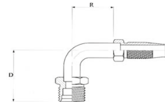
"O" ring buitendraad, 90° gebogen Male insert "O" ring, 90° elbow Raccord mâle "O" ring, coudé 90°
