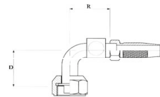
"O" ring wartel, met kijkglas, 90° gebogen "O" ring female swivel, with sight glass, 90° elbow "O" ring femelle tournant, avec "sight glass", coudé 90°
