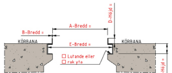
Figur 4. Smörjgrop
